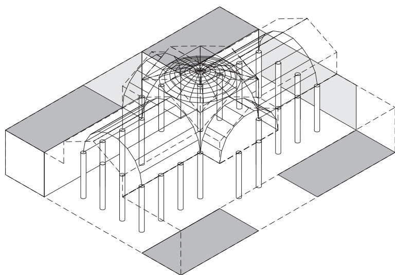
Casa França Brasil (Centro / Rio de Janeiro) — Arquiteto Grandjean de Montigny
