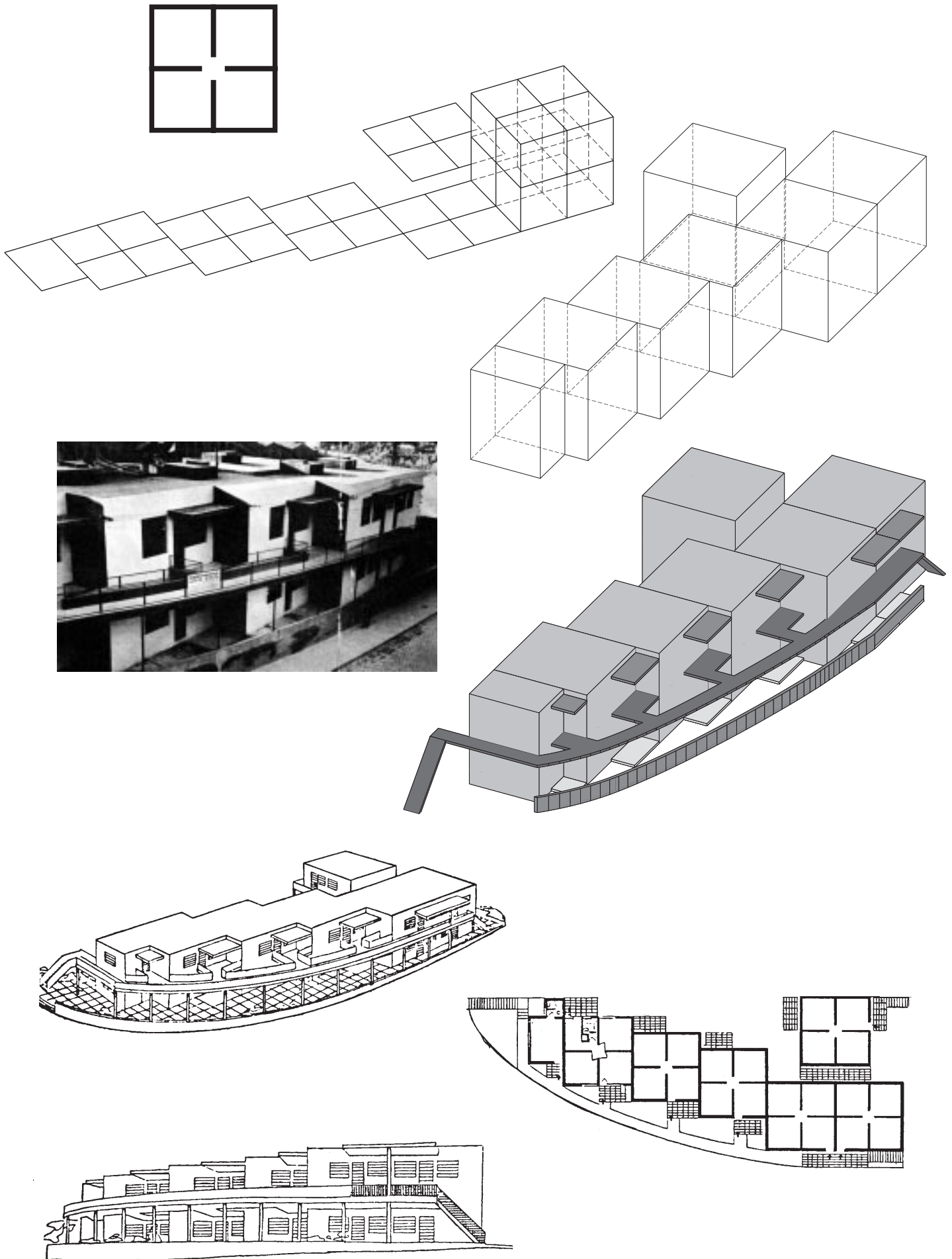
Habitação popular multifamiliar (Gamboa / Rio de Janeiro) —Arquiteto Lucio Costa
